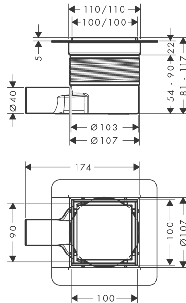
Maßzeichnung
