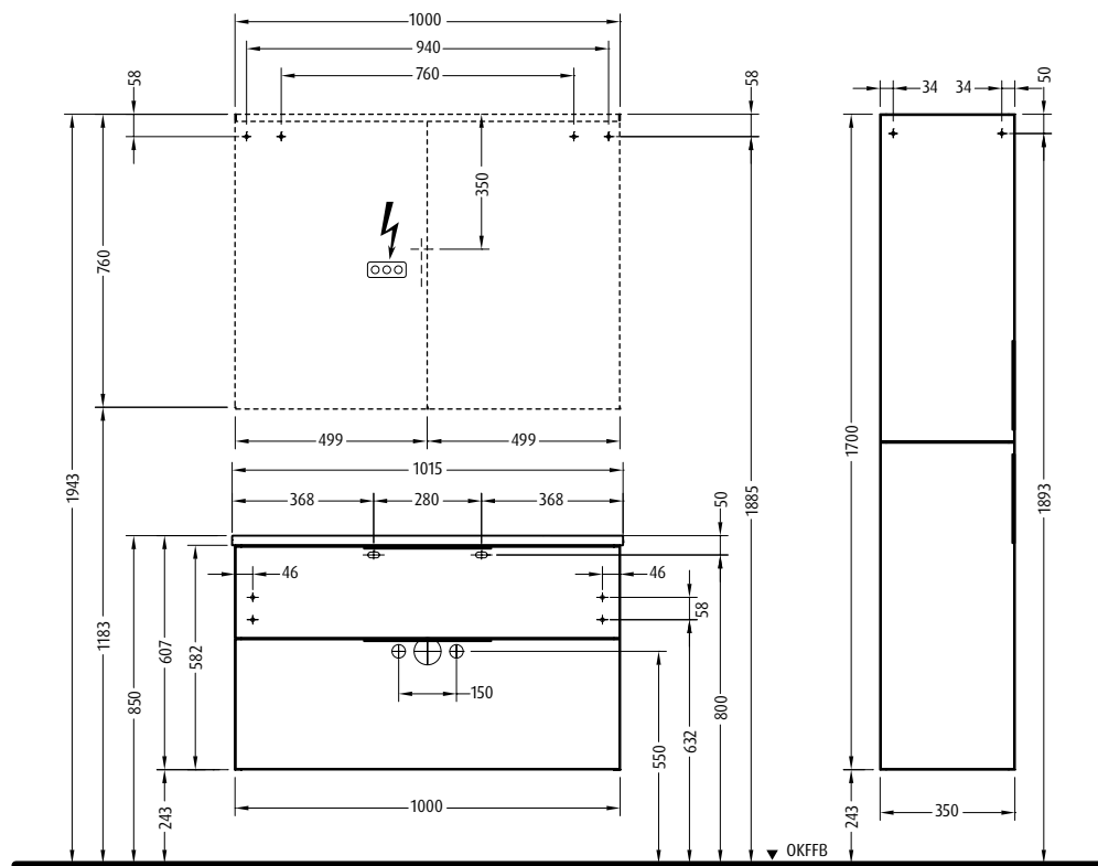
N L 220 - 240 V loser Netzanschluss (laut VDE 0100 Teil 701)
