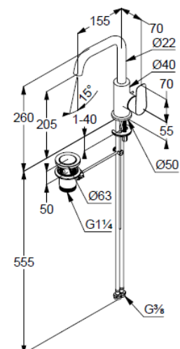
Maßzeichnung/ Dimensional drawing
