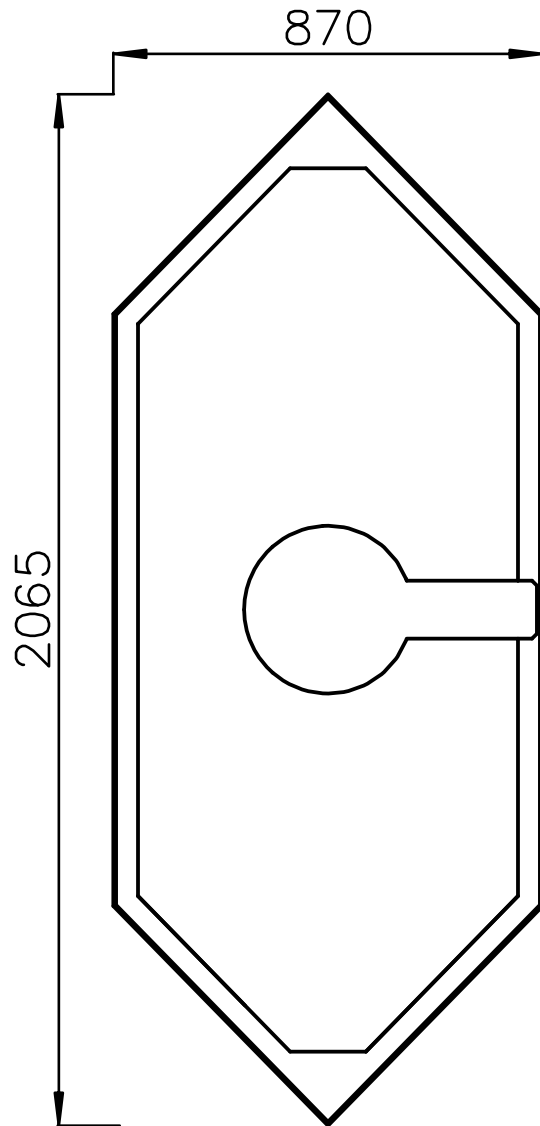
Draufsicht
