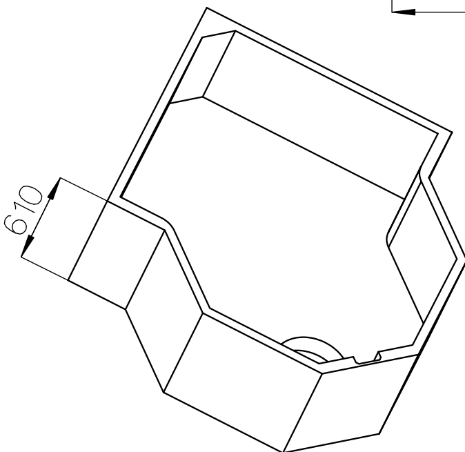
Isometrische Ansicht
