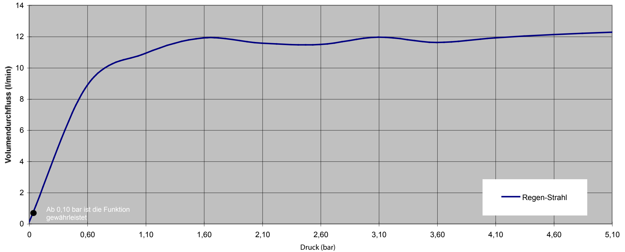
Durchflussdiagramm: Handbrause Nikles Stilo Quadro
