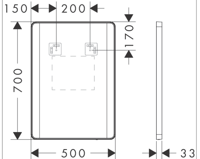
Maßzeichnung
