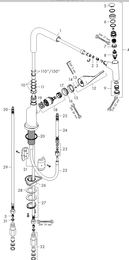
製品分解図
