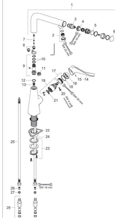
製品分解図
