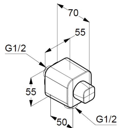
Maßzeichnung
