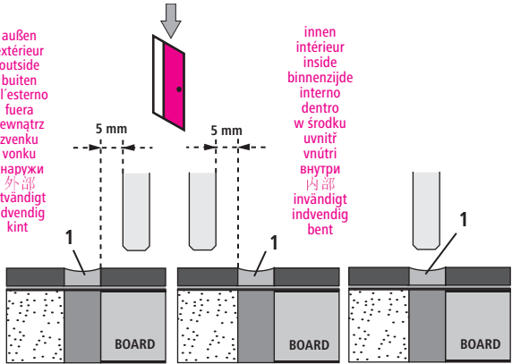
2 Versiegelung / Scellement / Sealing / Siliconen-kitnaad / Sigillatura / Sellado / Uszczelnienie zewnętrzne / Uzavirací náter / Tesniaca hmota / Герметик / 密封胶 / Försegling / Forsegling / Etazárs
