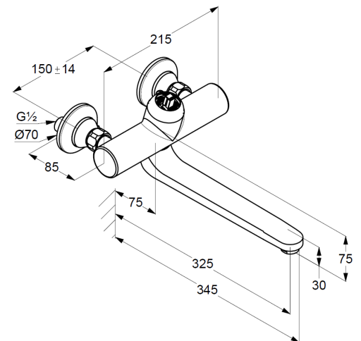
Maßzeichnung/ Dimensional drawing
