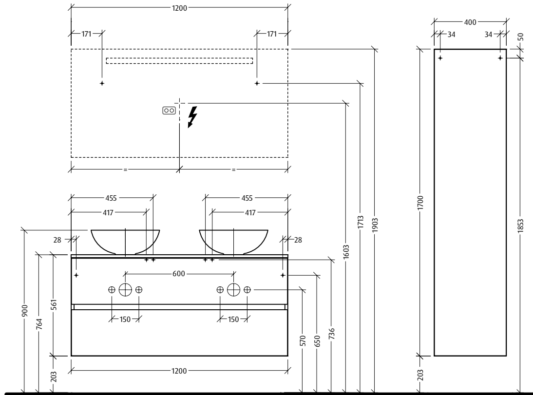
NL 220 - 240 V geschalteter Netzanschluss (laut VDE 0100 Teil 701)
