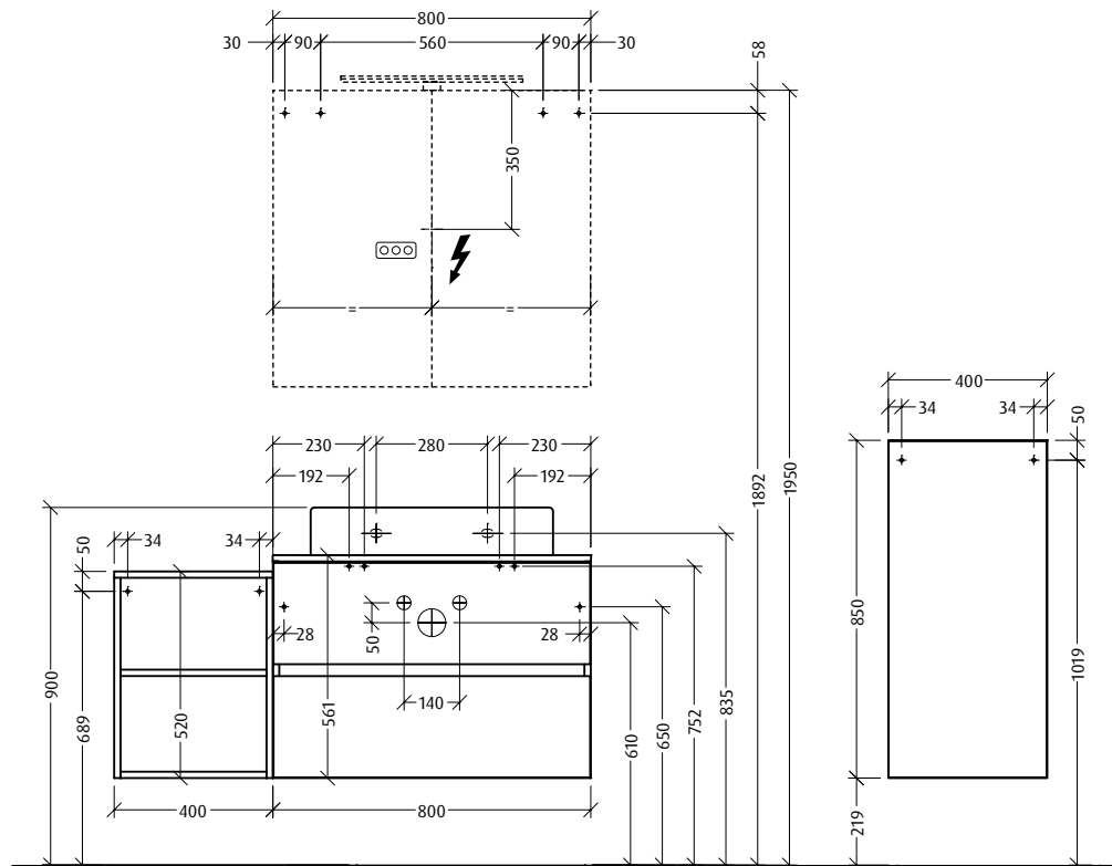
N=L 220 - 240 V loser Netzanschluss (laut VDE 0100 Teil 701)
