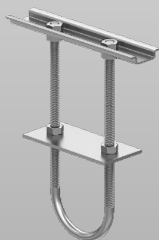
Fensterbankträger für Radiatoren
