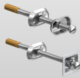
Halter zu Mauerkonsole
