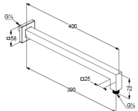
Maßzeichnung/ Dimensional drawing
