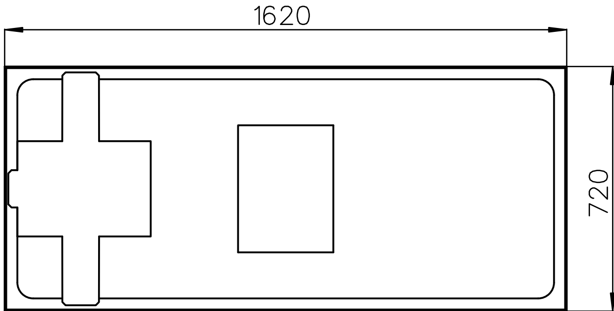
Draufsicht
