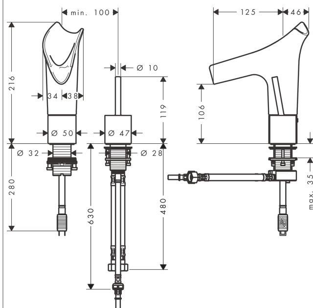
Maßzeichnung
